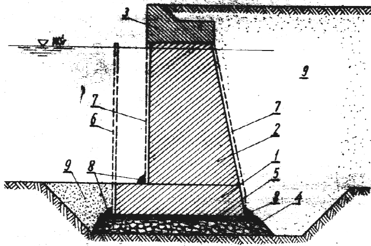
Rys. 5.65. Nabrzeże monolityczne wykonane pod wodą 1 - fundament wykonany pod wodą, 2 - konstrukcja podwodna wykonana pod wodą, 3 - nadbudowa wykonana na sucho, 4 - podsypka kamienna, 5 - warstwa wyrównująco uszczelniająca, 6 - deskowanie fundamentu (usunięte po jego wykonaniu), 7 - deskowania części podwodnej nabrzeża, 8 - uszczelnienia deskowań z worków z betonem, 9 - zasyp po wykonaniu nabrzeża
