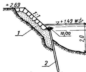
Rys. 5.74. Przekrój podrzędny nabrzeża ze ścianką szczelną wolno stojącą 1 — żwir, 2 — ścianka szczelna drewniana z brusów 12/30 cm, 3,5 m dl.
