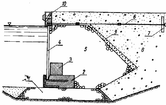
Rys. 5.70. Nabrzeże tarczowe [12]
