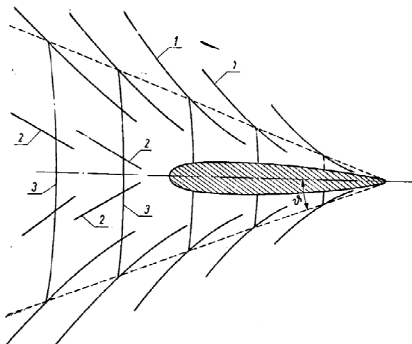
Rys. 3.65. Układ fal okrętowych w czasie ruchu statku w basenie o głębokiej wodzie [71]
