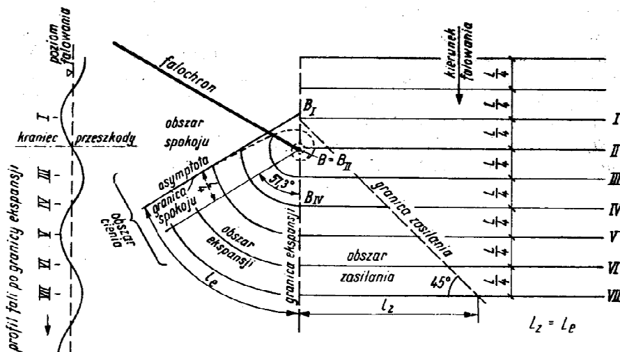
Rys. 3.31. Plan falowania z uwzględnieniem dyfrakcji metodą Iribarena
